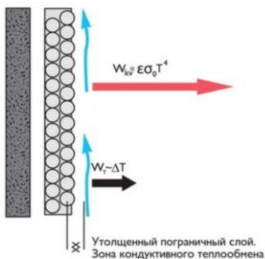
Рис.6. Иллюстрация механизмов теплоотдачи от поверхности теплоизоляции КОРУНД
